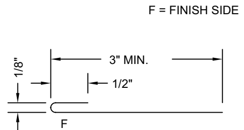
J-CLIP
